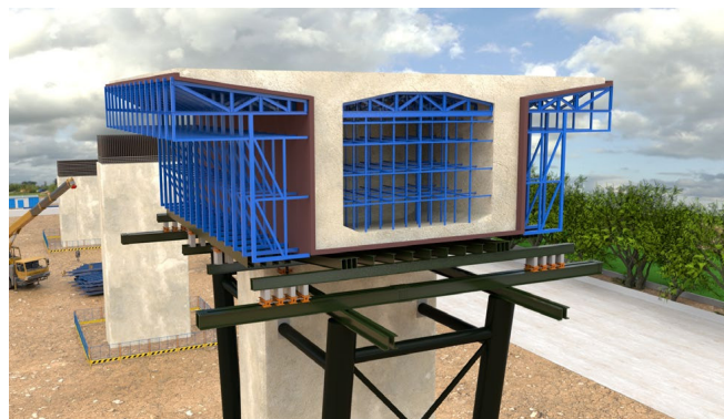
侧模板落架
