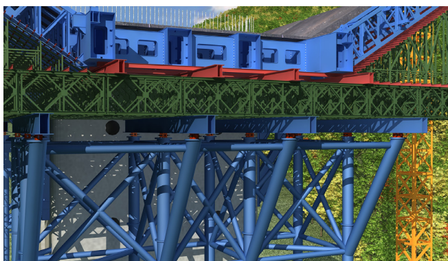
落地钢支架
