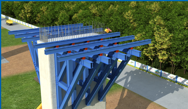
三角托架
